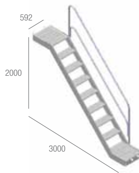
16. ESCALERA DE VISTA 8 PELDAÑOS CONSOLE BRACKET ESCALIER VISITEUR À 8 ÉCHELONS
