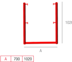
11. PIE BARANDILLA DOBLE DOUBLE HANDRAIL FOOT PIED GARDE-CORPS 2 CÔTES
