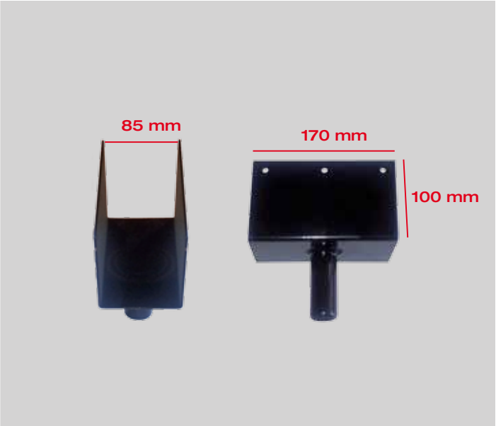
Cabezal sencillo / Simple head / Fourche simple
