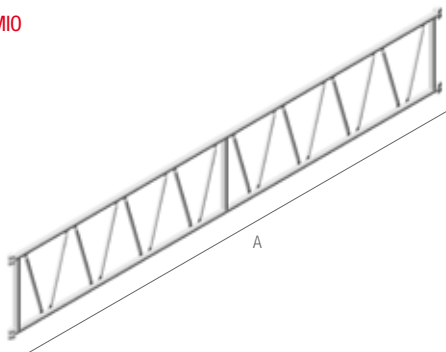
18. LARGUERO REFORZADO DOUBLE LEDGER POUTRELLE REINFORCÉE
